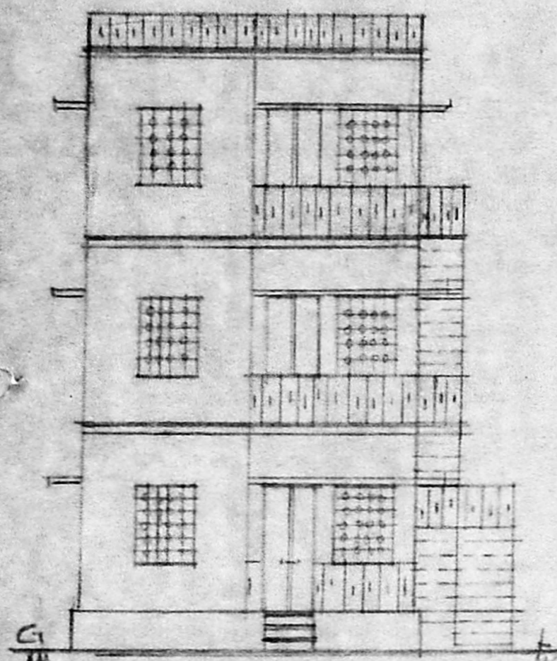
ELEVATION
